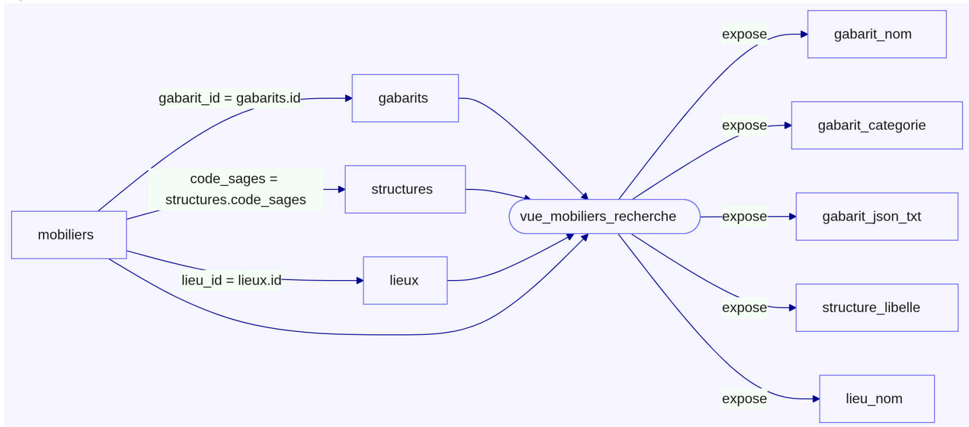
Diagramme — Jointures de la vue vue_mobiliers_recherche
