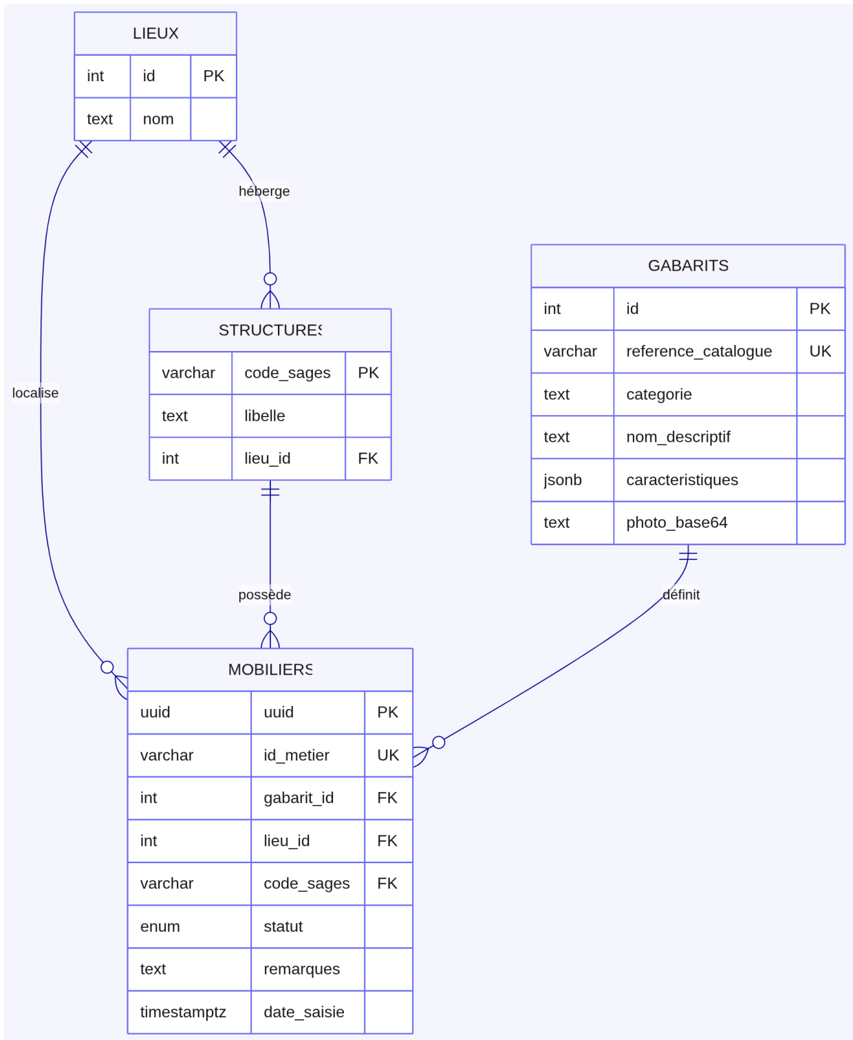
Diagramme — Modèle Conceptuel de Données (MCD / ERD)
